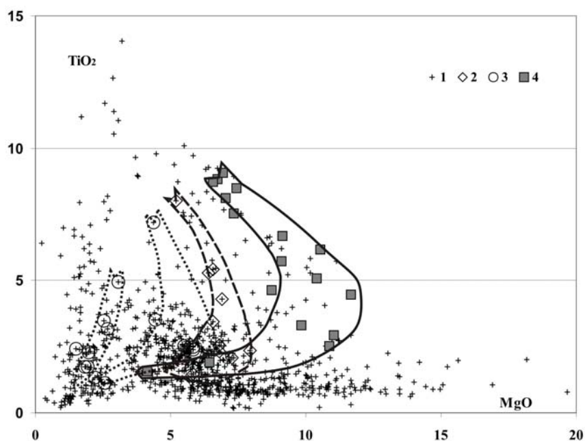
Рис. 1. Диаграмма \text{TiO}_2 – \text{MgO} пород Чинейского массива и макроритма 1Т. 1- Общая выборка, 2-4 – макроритм 1Т: 2-ритмы 560-562 м, 3-ритмы 384-532 м, 4-микроритмы 622 м.
